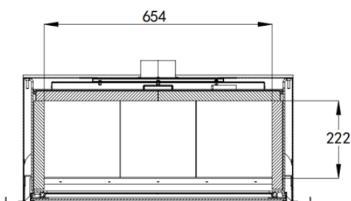
B-B
